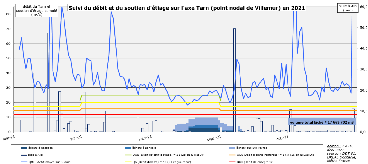
Figure 1 : suivi du débit et du soutien d'étiage sur le Tarn au point nodal de Villemur-sur-Tarn entre le 1er juin et le 31 octobre 2021. CA 81, 2021
